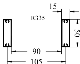
Detalhe Perfil R335
