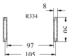
Detalhe Perfil R334
