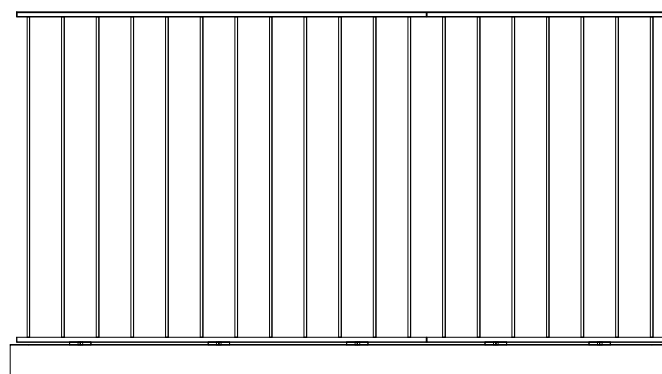
Detalhe Perfil R334
